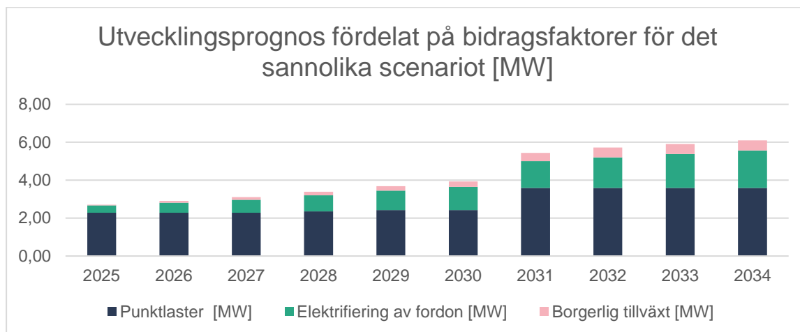
Figur 4 Det sannolika prognoss scenariot uppdelat på bidragande faktorer. Det är tydligt att den dominerande faktorn i prognosen är punktlasterna.
